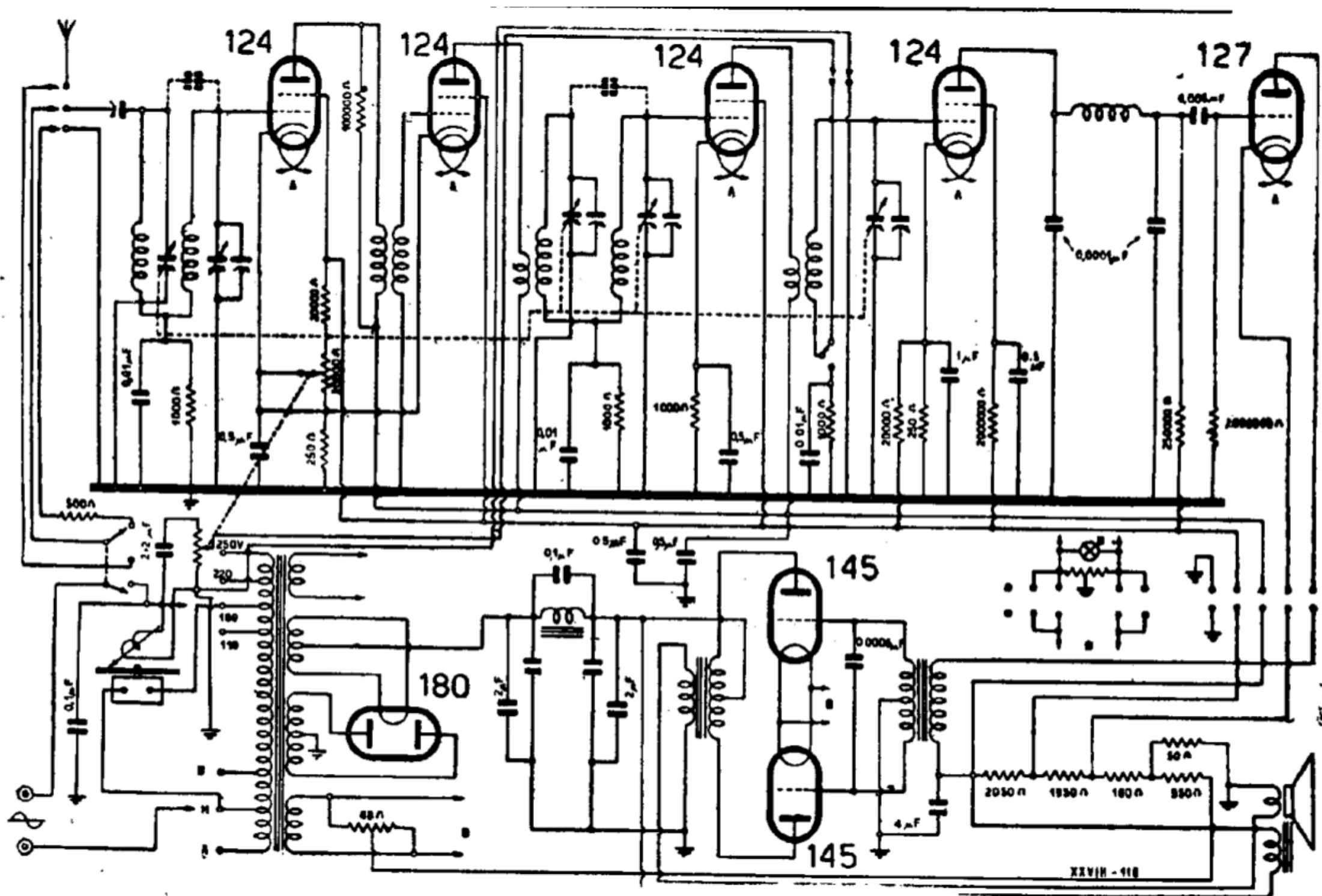
RADIOMARELLI - MOD. « CHILIOFONO I »
